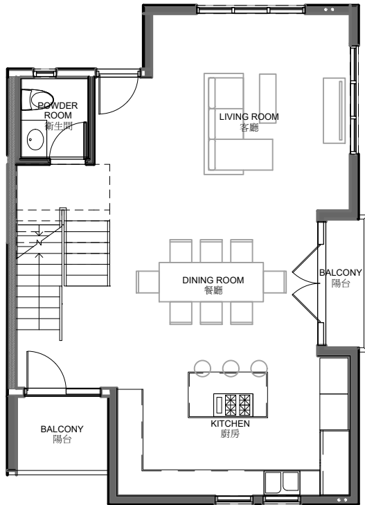
First Floor Plan 904 S.F. 一樓平面圖
